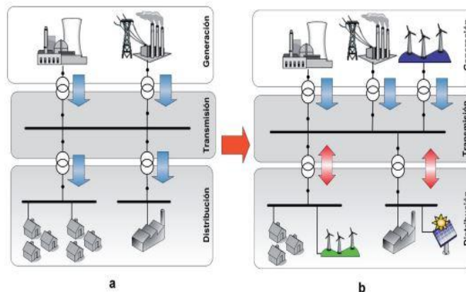
Fig. 1. Sistemas de energía eléctrica (a) tradicional y (b) próxima generación (Diaz & Hernández, 2015)
